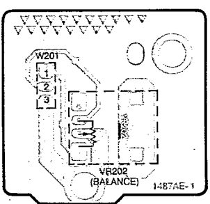
D BALANCE VR. P.C.B. (REP2156A-2S)
